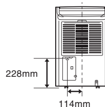
連續排水孔位置
